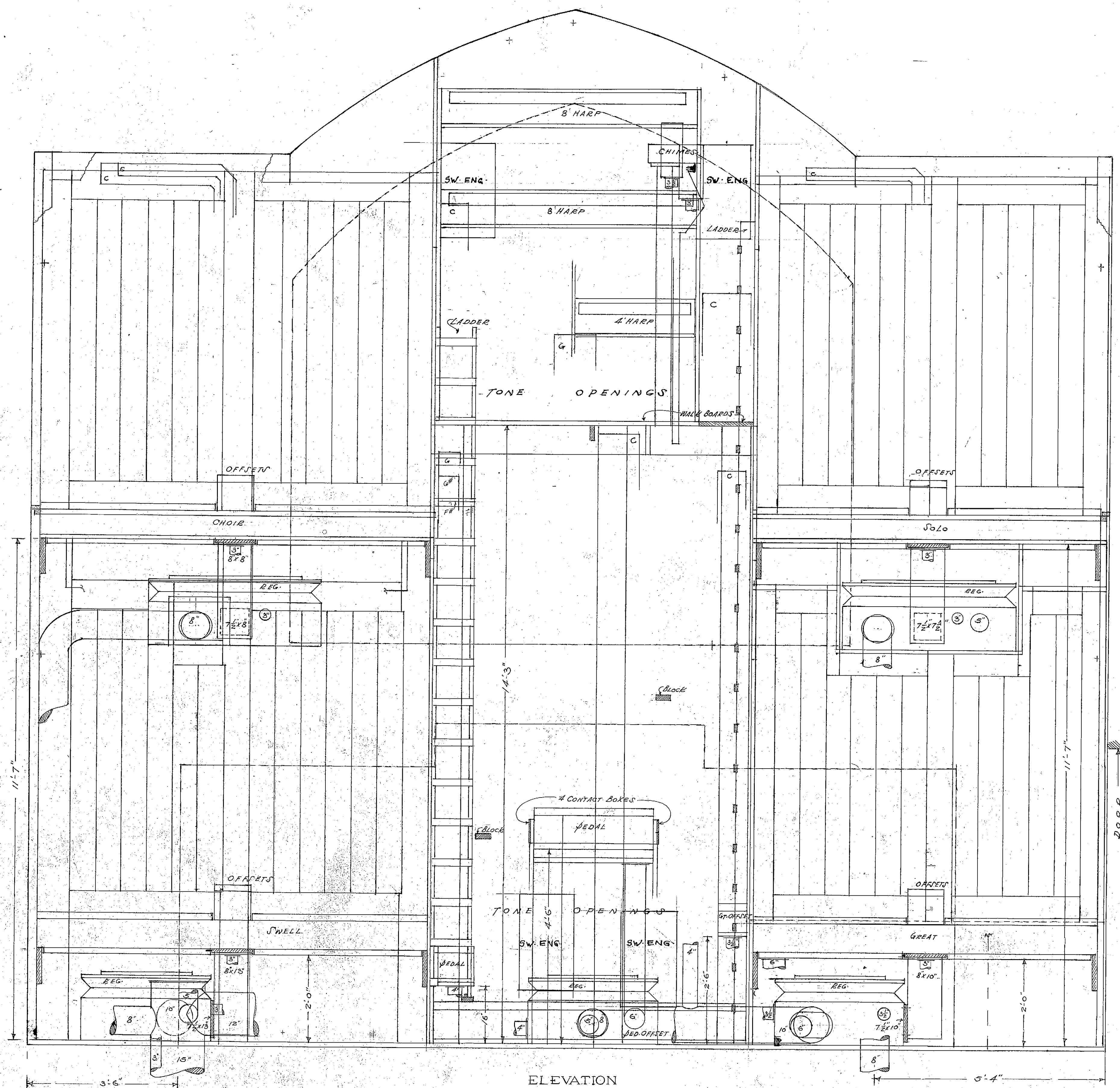
ELEVATION
