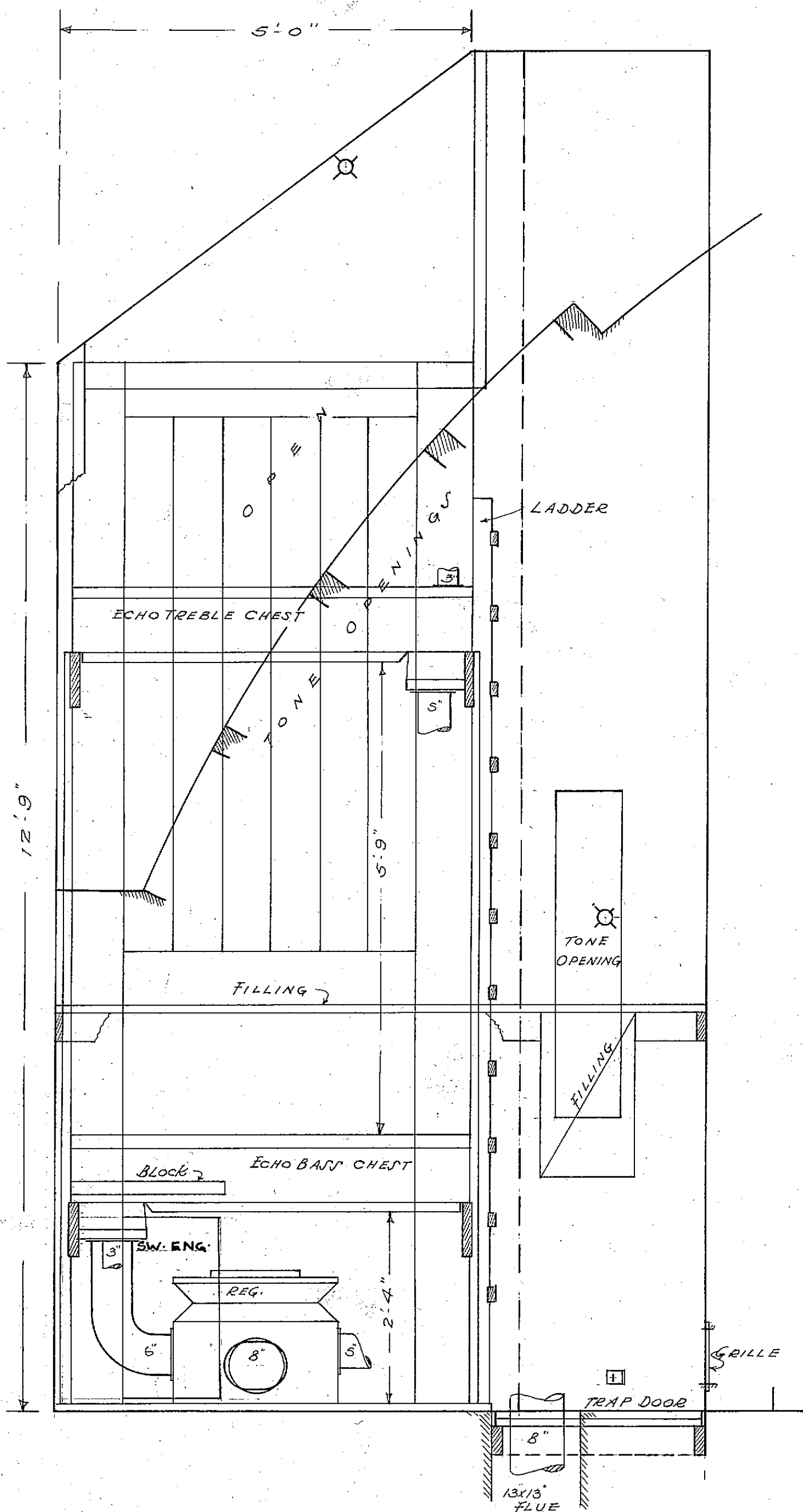
ELEVATION
