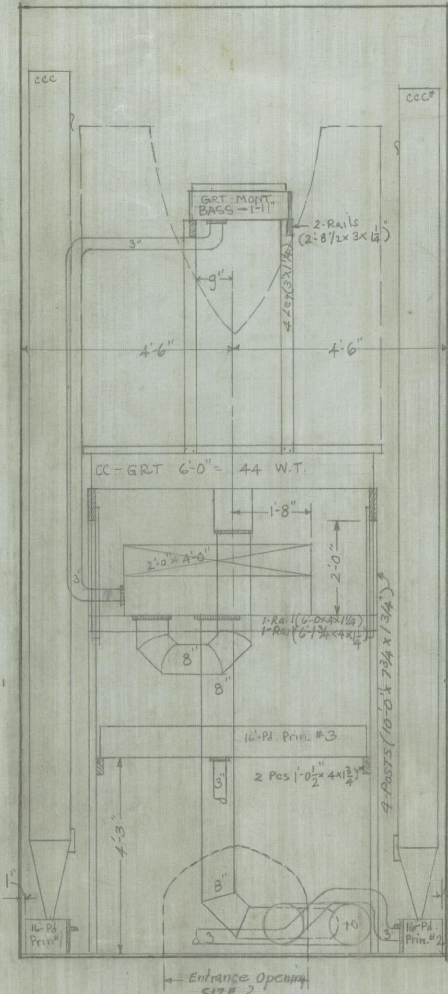
ELEVATION B-B
