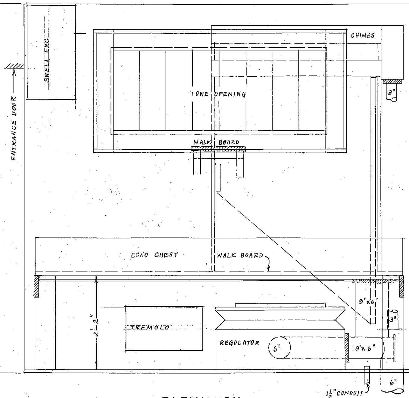
ELEVATION
