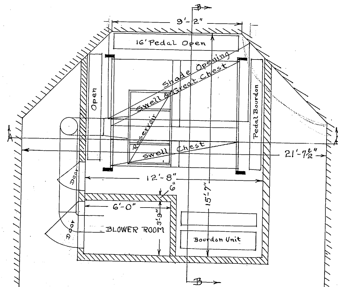
PLAN Scale-1/4"=1'-0"
