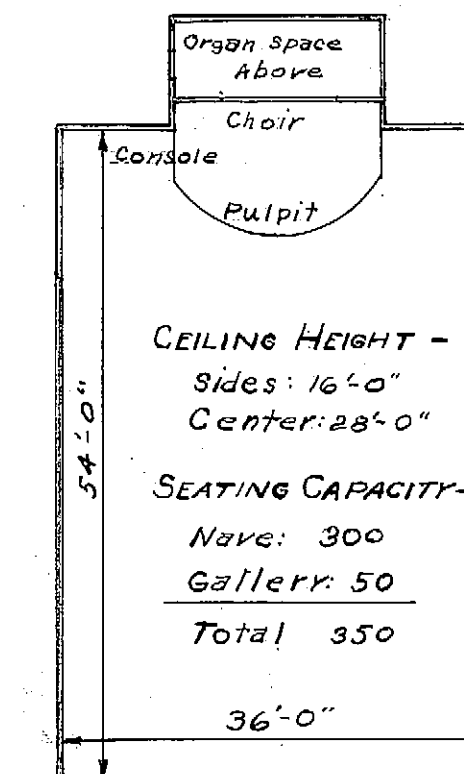
AUDITORIUM PLAN Scale: 1/8" = 1'-0"
